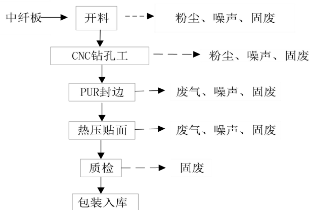
图 2.2-2 项目生产工艺流程及产污环节图
