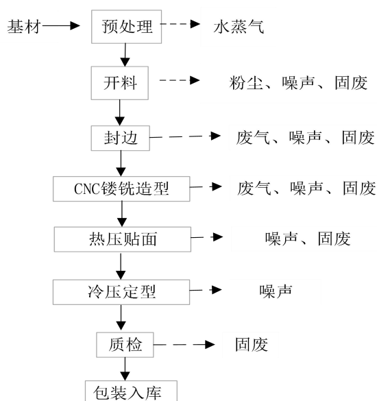
图 2.2-2 项目生产工艺流程及产污环节图
